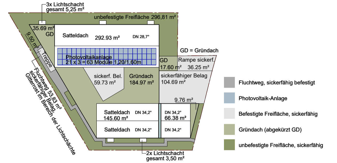
DACHAUSICHT / BEFESTIGTE FLÄCHEN 1:500
