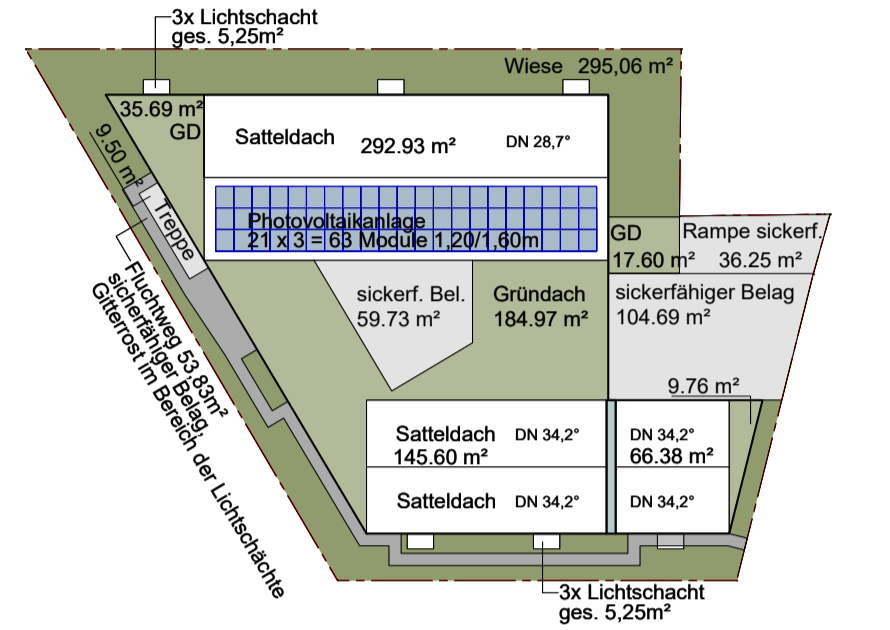
DACHAUSICHT / BEFESTIGTE FLÄCHEN 1:500
