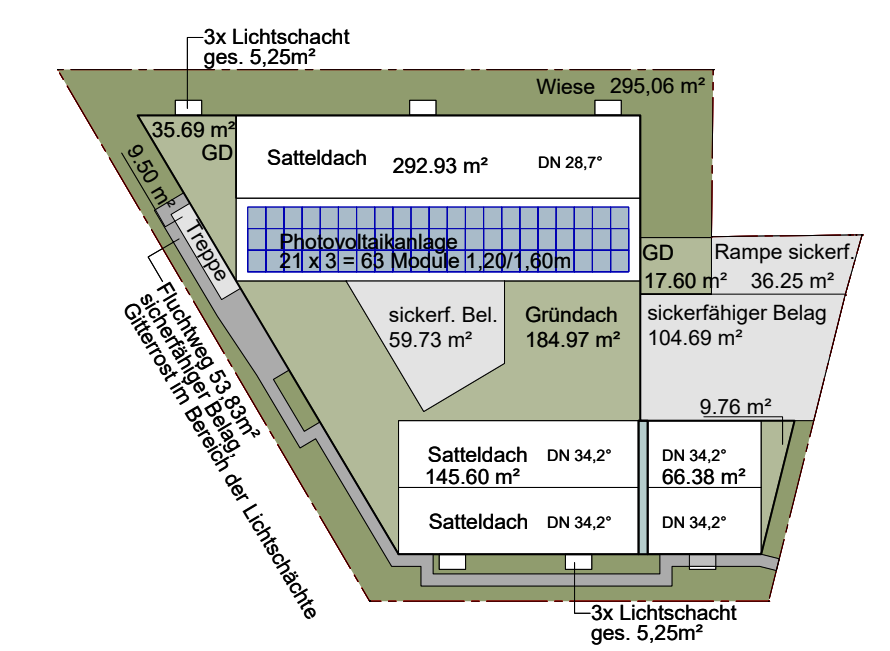
DACHAUFSICHT / BEFESTIGTE FLÄCHEN 1:500
